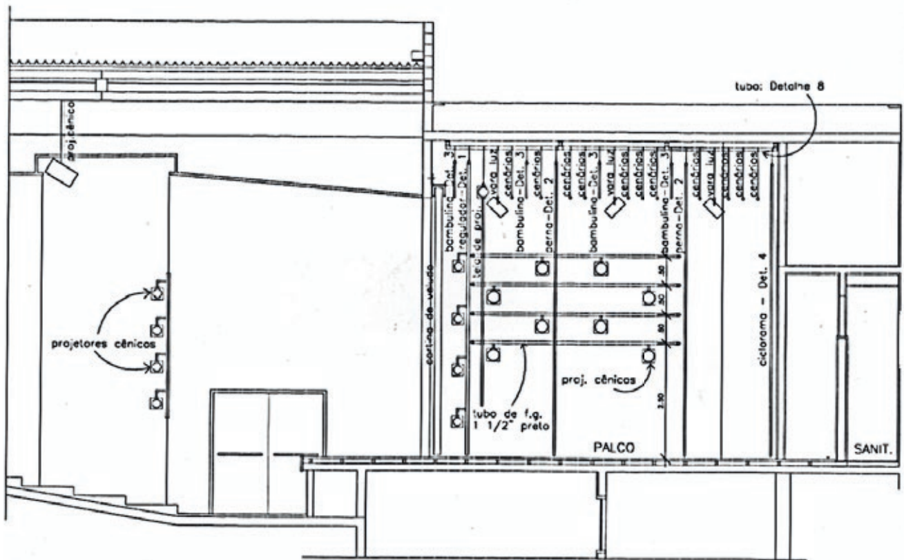
1 UC-01 CORTE AA ESCALA 1:50
